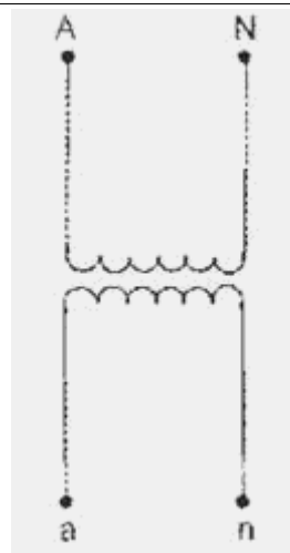
Slika 2 Oznake priključaka naponskih mernih transformatora
