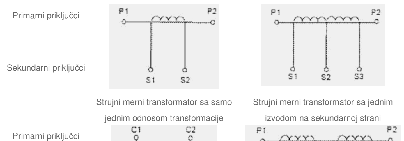
Slika 1 Oznake priključaka strujnih mernih transformatora
