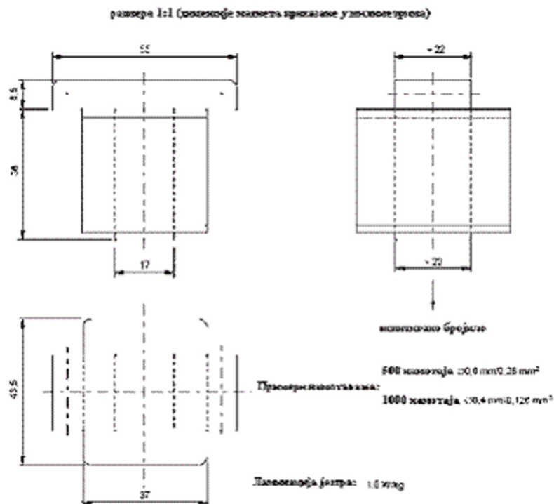
Slika 3 - Specifikacija elektromagneta
