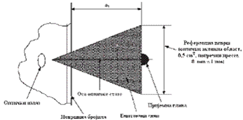
Slika 1 - Optički izlaz za ispitivanje
