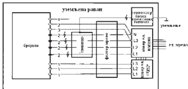
Slika 5 - Ispitivanje naponskih kola
