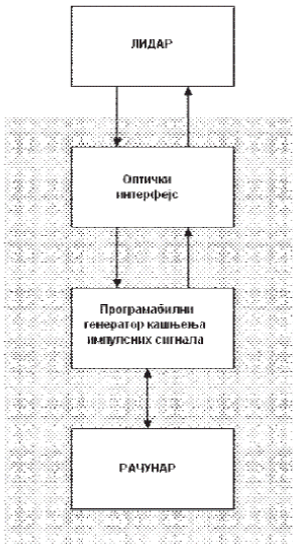
Slika 3 - Blok šema simulatora
